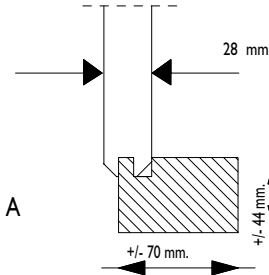
Zij aanzicht Seiten Ansicht Side view
