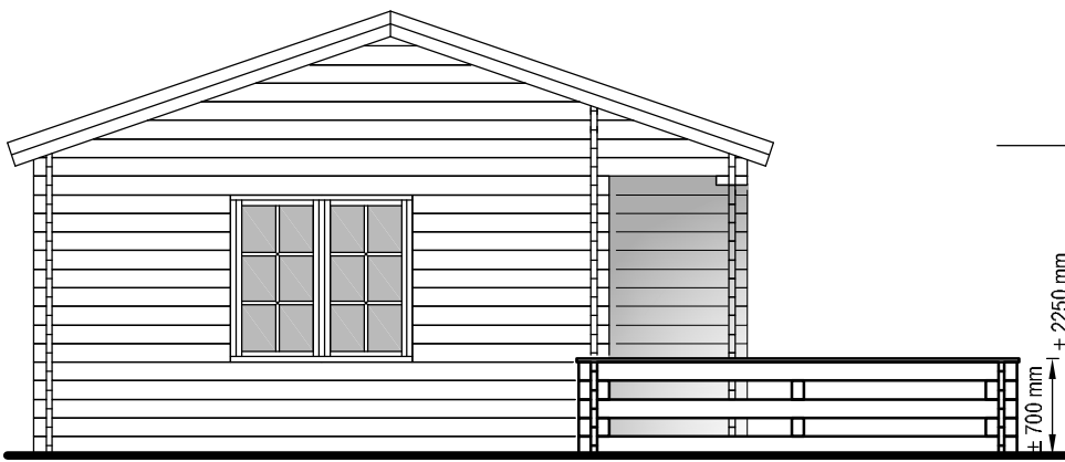
Voor aanzicht Vorder Ansicht Front view
