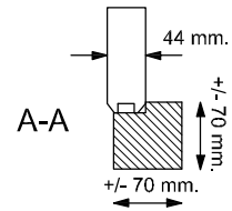
Voor aanzicht Vorder Ansicht Front view
