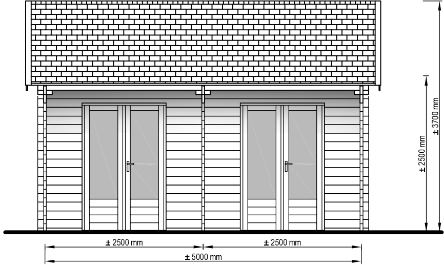
Zij aanzicht Seiten Ansicht Side view
