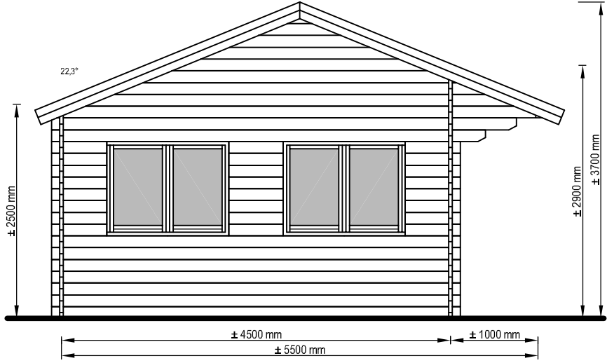
Voor aanzicht Vorder Ansicht Front view
